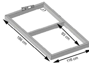
Betonstreifenfundament
