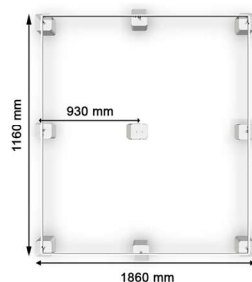
Punktfundament
